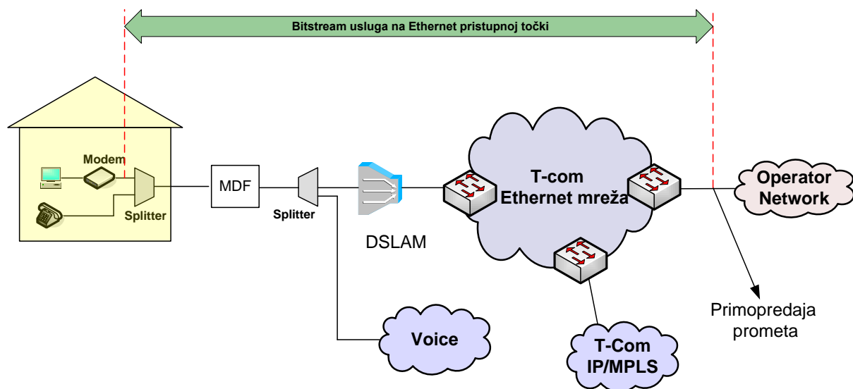
Slika 14. Veleprodajni širokopolasni pristup za pružanje VoIP usluge na Ethernet razini u slučaju kada Krajnji korisnik ostvaruje Osnovni pristup mreži putem usluge T-Coma
