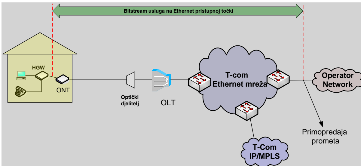
Slika 5. Veleprodajni širokopoljasni pristup za pružanje Internet usluge na Ethernet razini kod pristupa preko FTTH rješenja
