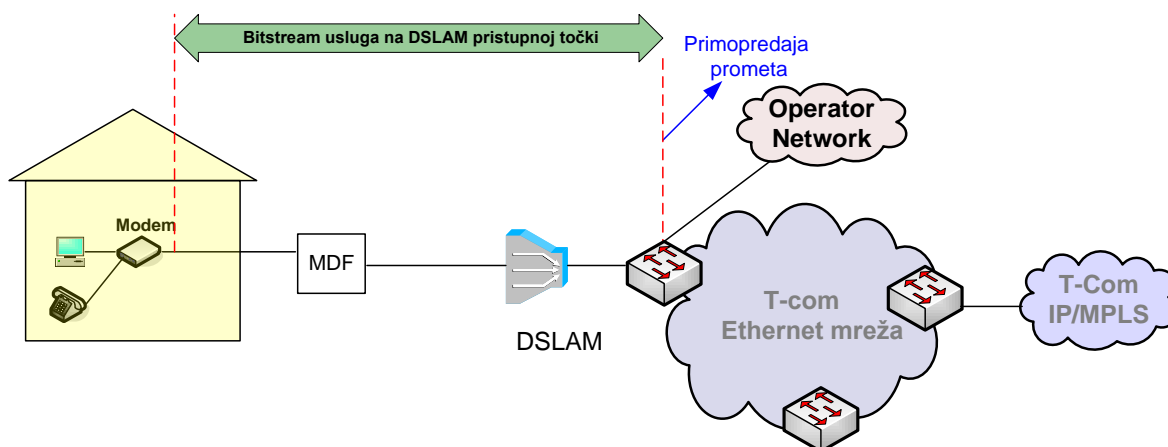
Slika 7. Veleprodajni širokopoljasni pristup za pružanje Internet usluge na DSLAM razini u slučaju kada Krajnji korisnik ostvaruje Osnovni pristup mreži putem usluge T-Coma
