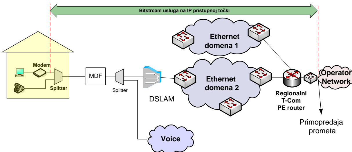
Slika 16. Veleprodajni širokopolasni pristup za pružanje VoIP usluge na IP razini u slučaju kada Krajnji korisnik ostvaruje Osnovni pristup mreži putem usluge T-Coma
