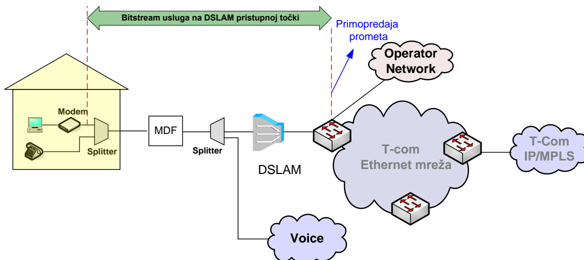
Slika 7. Veleprodajni širokopoljasni pristup za pružanje Internet usluge na DSLAM razini u slučaju kada Krajnji korisnik ostvaruje Osnovni pristup mreži putem usluge T-Coma
